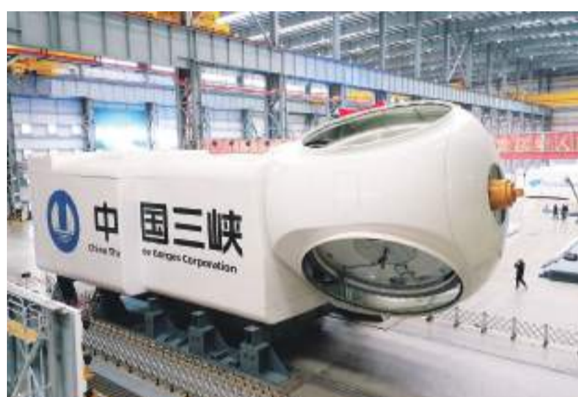
11月23日在福建三峡海上风电国际产业园下线的16兆瓦海上风电机组(无人机照片)。林善传/图
