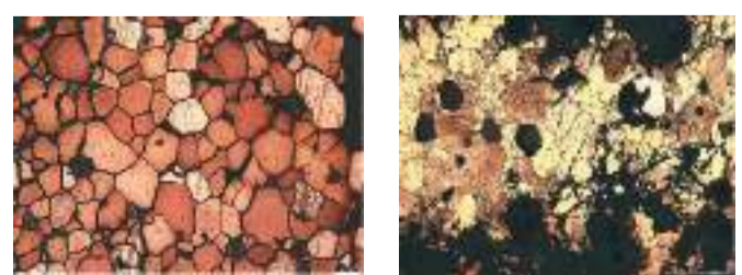
通过现代扫描技术从三星堆神树等器物中发现了使用销杆和铆钉等机械连接结构，并在神树中发现了芯骨的使用。 对三星堆神树组件结构进行扫描看到的金相。 三星堆神树组件芯骨部分的金相则是另外一种模样。
