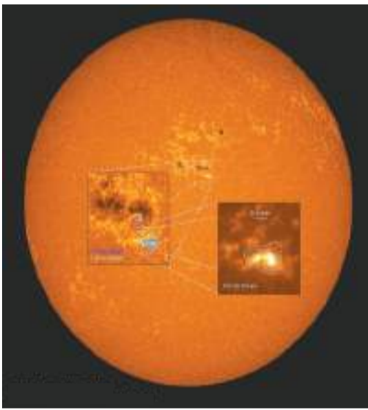
圖為「夸父一號」太陽硬X射線成像儀（HXI）在2022年11月11日觀測到的一個C級耀斑硬X射線成像與AIA/SDO紫外1700圖像的比較。 中新社
