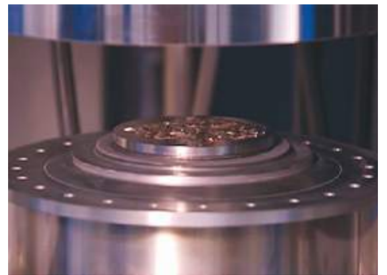
CVD法人工培育钻石的培养舱。
