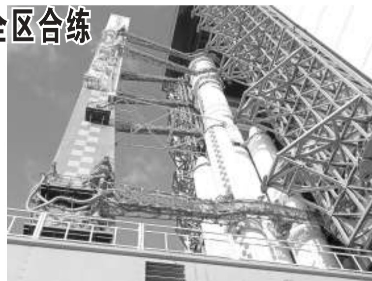
1月15日，天舟七号货运飞船与长征七号遥八运载火箭组合体开始转运。当日，天舟七号货运飞船与长征七号遥八运载火箭组合体垂直转运至发射区。
